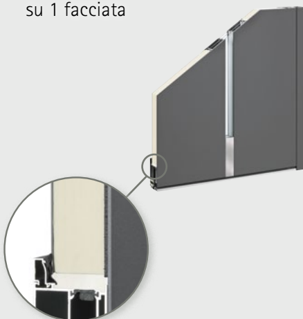
Pannello applicato su 1 facciata
